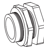
Adaptador Especial 2" Y 3" Para tanques de 5.000 L, 10.000 L, 15.000 L y 20.000 L.
